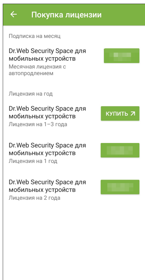
Рисунок 3. Покупка лицензии
