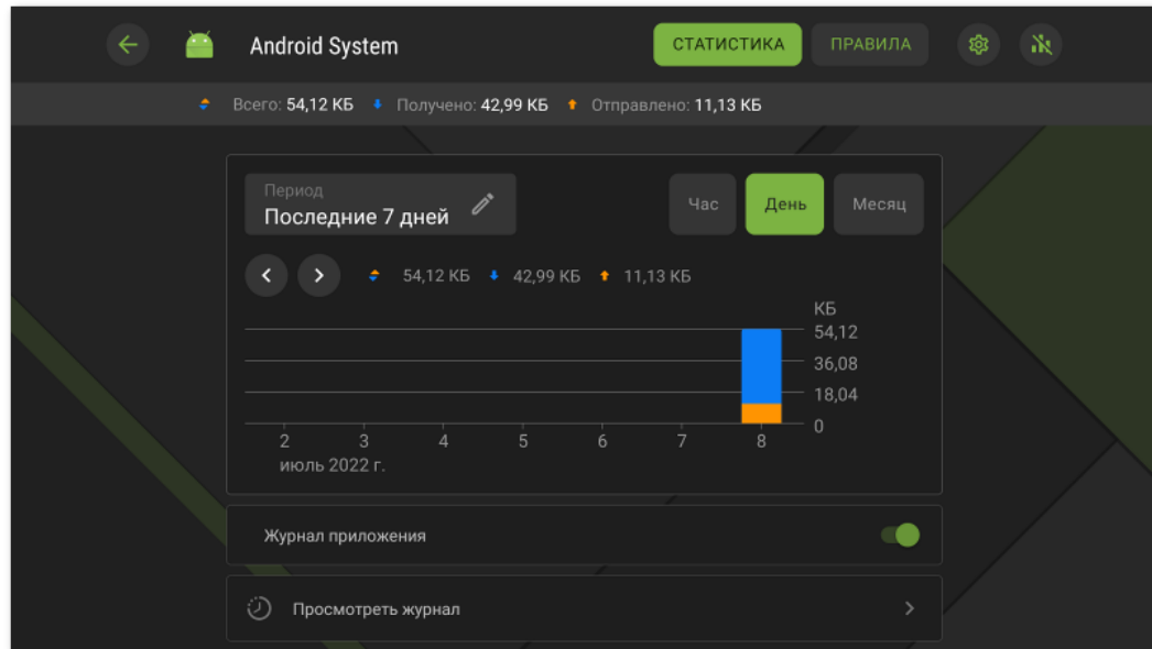
Рисунок 40. Экран приложения
