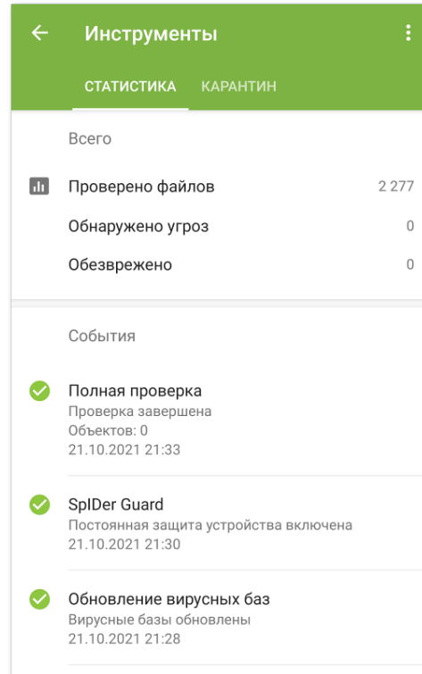
Рисунок 32. Статистика
