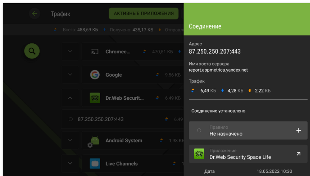
Рисунок 42. Экран Соединение
