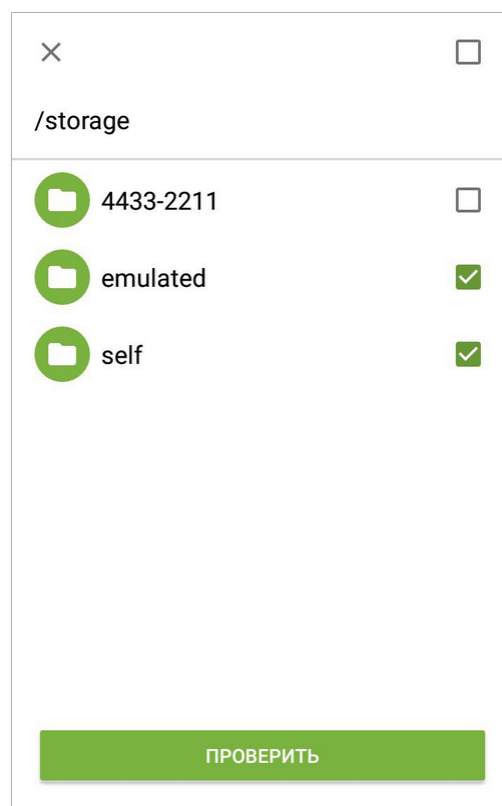
Рисунок 15. Выборочная проверка
