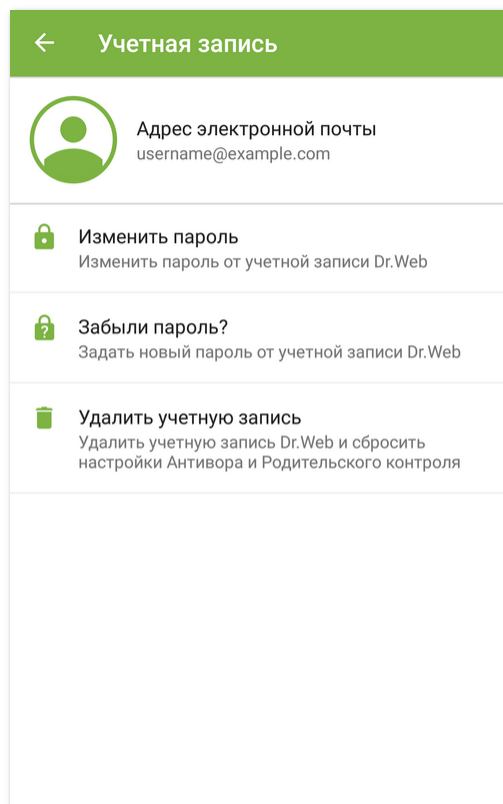
Рисунок 12. Учетная запись
