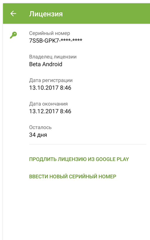
Рисунок 6. Продление лицензии
