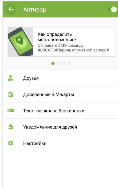
Рисунок 18. Антивор Dr.Web
