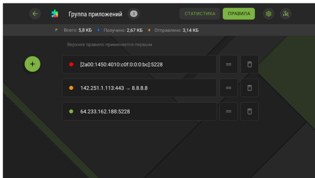
Рисунок 43. Вкладка Правила
