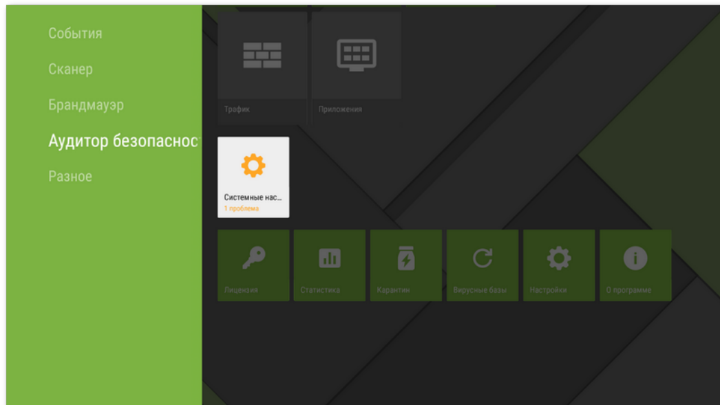
Рисунок 45. Аудитор безопасности
