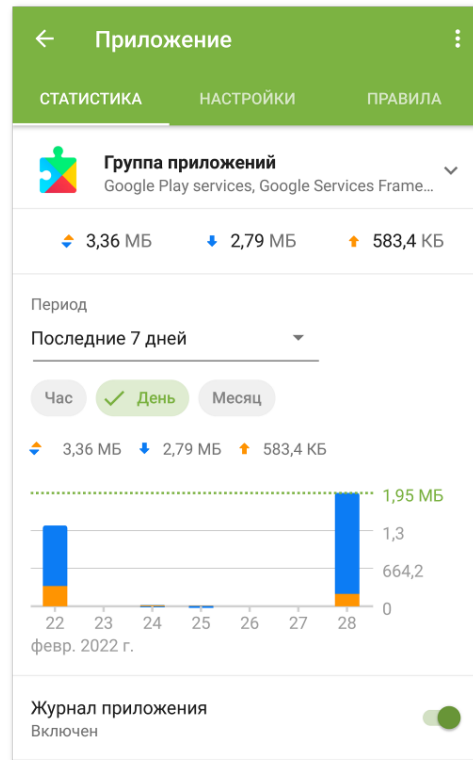
Рисунок 28. Экран Приложение
