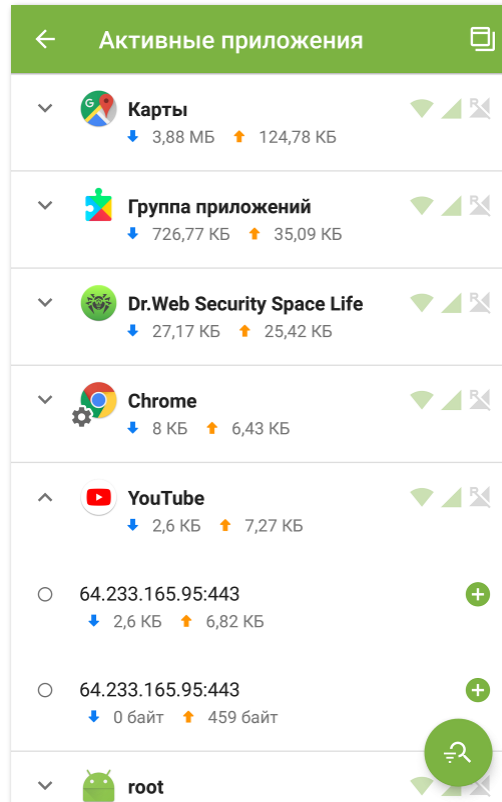
Рисунок 24. Активные приложения
