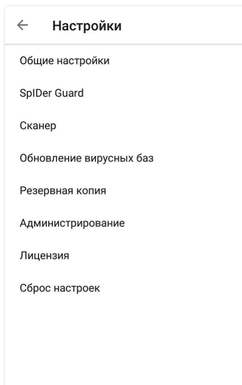
Рисунок 34. Настройки
