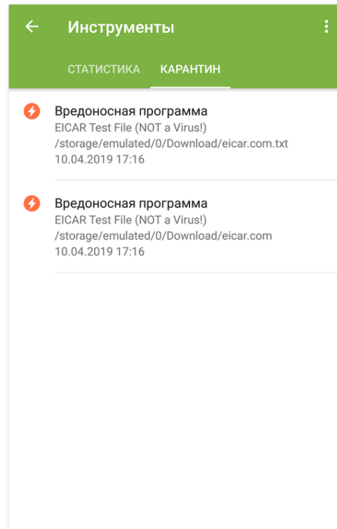
Рисунок 33. Карантин
