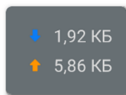
Рисунок 25. Плавающее окно
