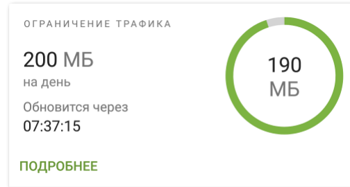
Рисунок 27. Ограничение трафика
