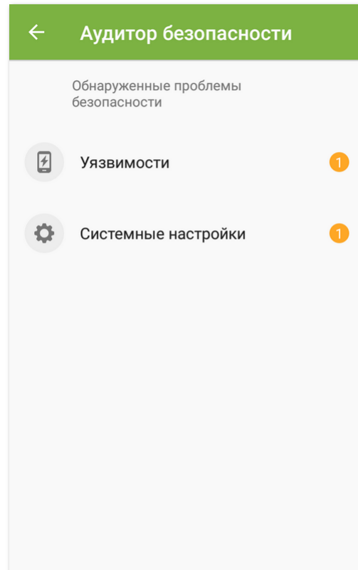
Рисунок 31. Аудитор безопасности
