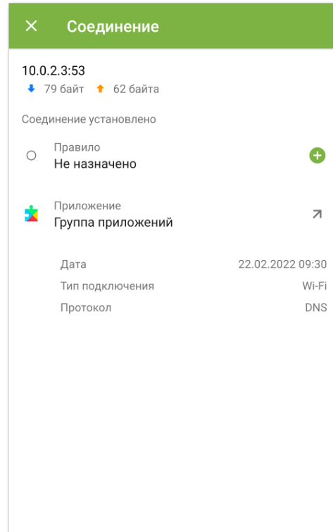
Рисунок 30. Экран Соединение
