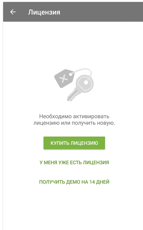
Рисунок 1. Экран Лицензия
