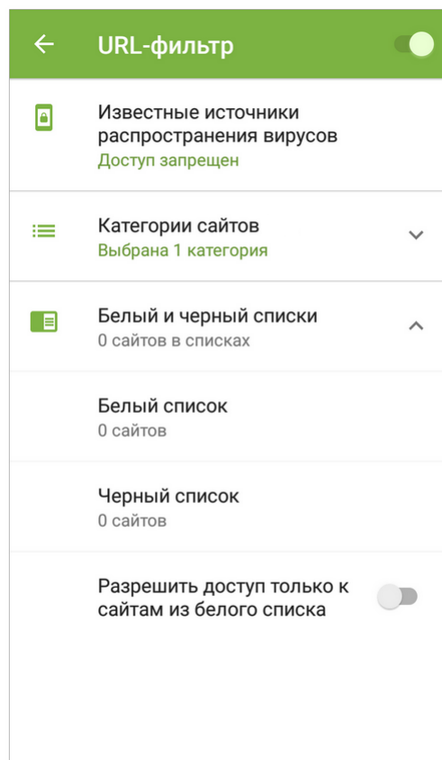
Рисунок 17. URL-фильтр
