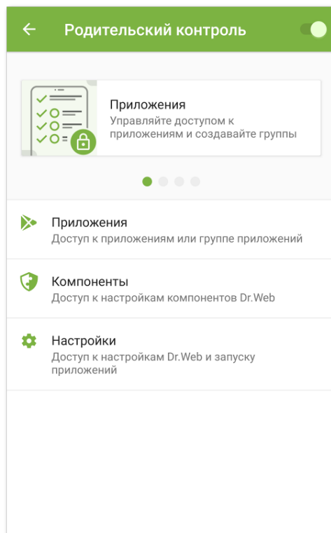
Рисунок 19. Родительский контроль
