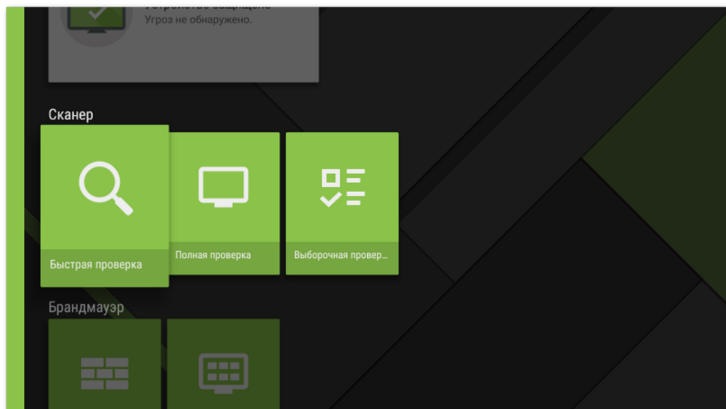
Рисунок 37. Сканер Dr.Web
