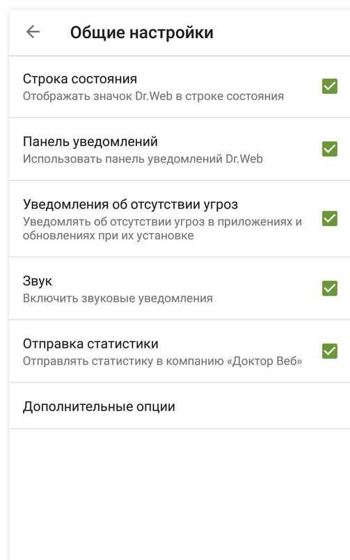
Рисунок 35. Общие настройки
