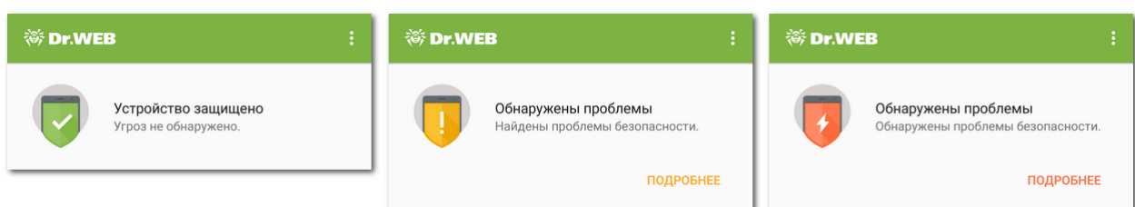
Рисунок 9. Панель состояния
