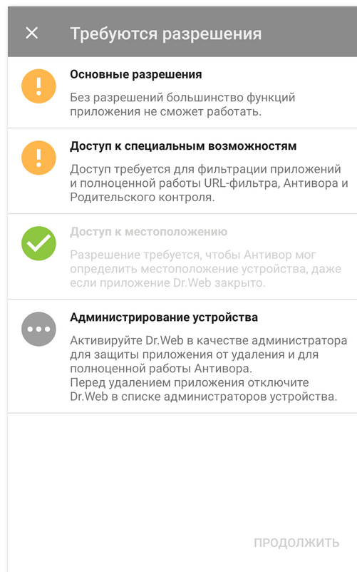
Рисунок 7. Требуются разрешения
