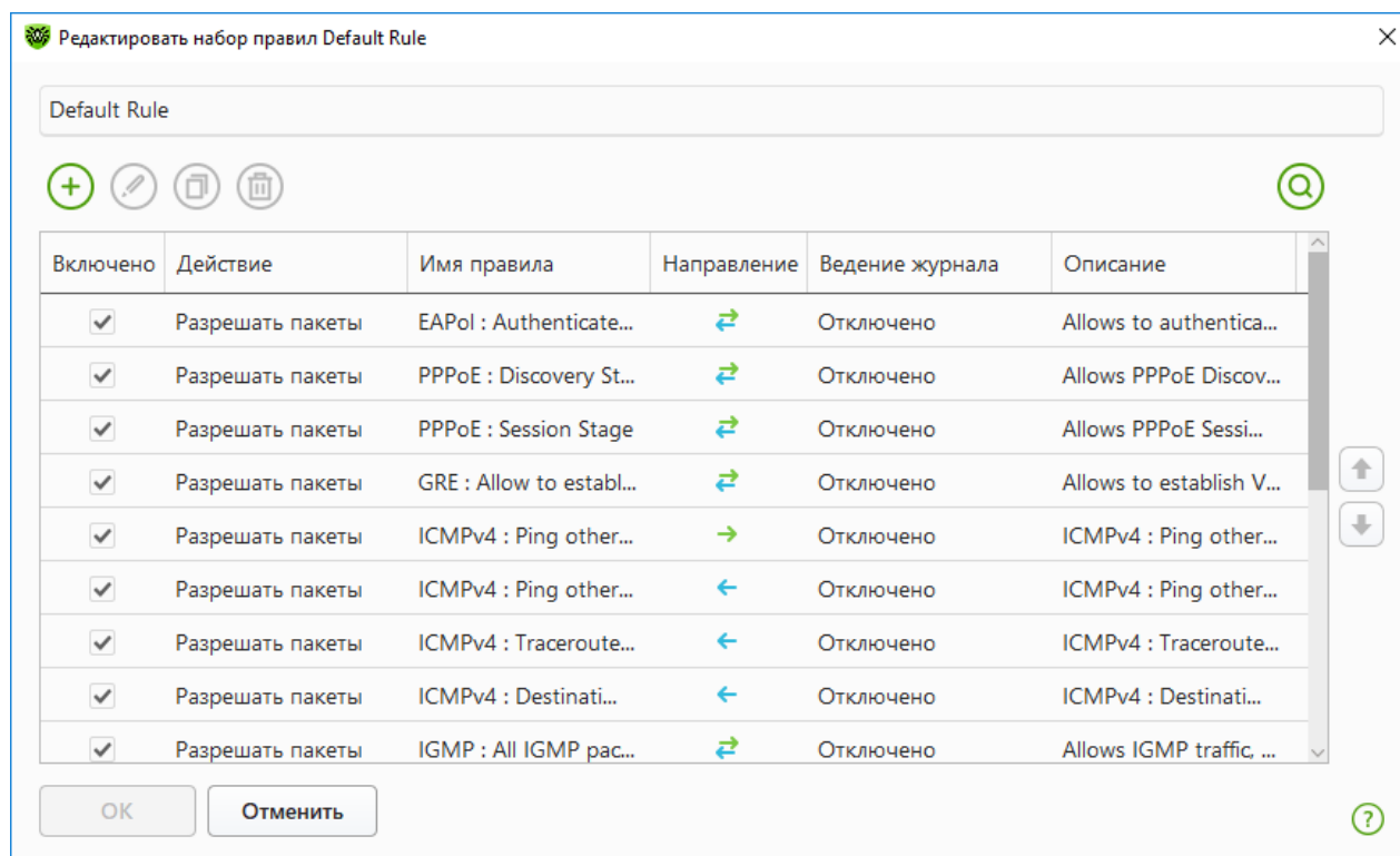
Рисунок 48. Набор правил фильтрации пакетов
