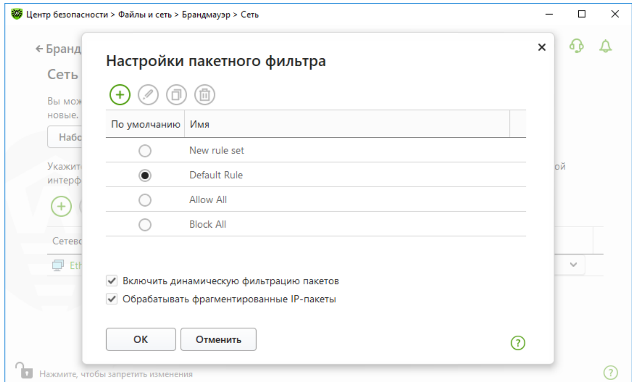
Рисунок 47. Окно Настройки пакетного фильтра
