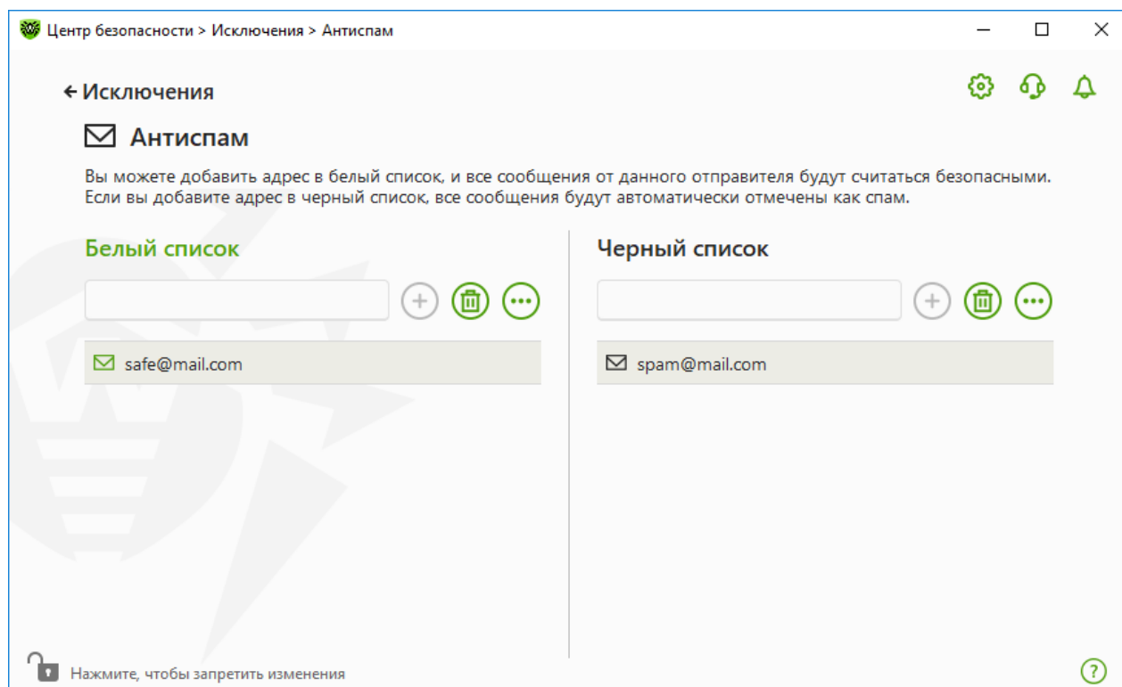
Рисунок 94. Черный и белый список адресов
