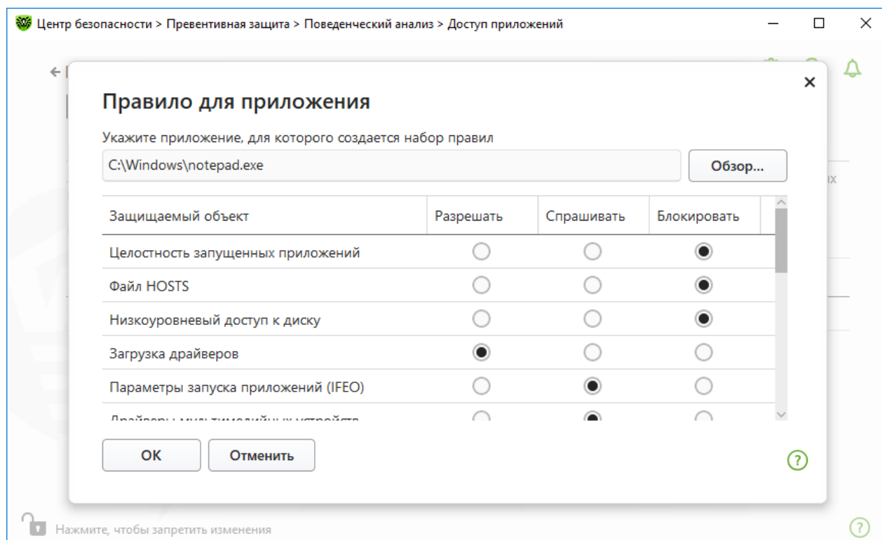
Рисунок 65. Добавление набора правил для приложения
