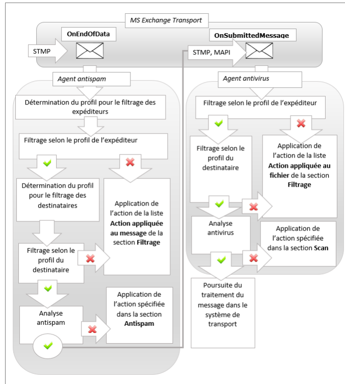
Schéma 1. Filtrage des messages dans le système de transport
