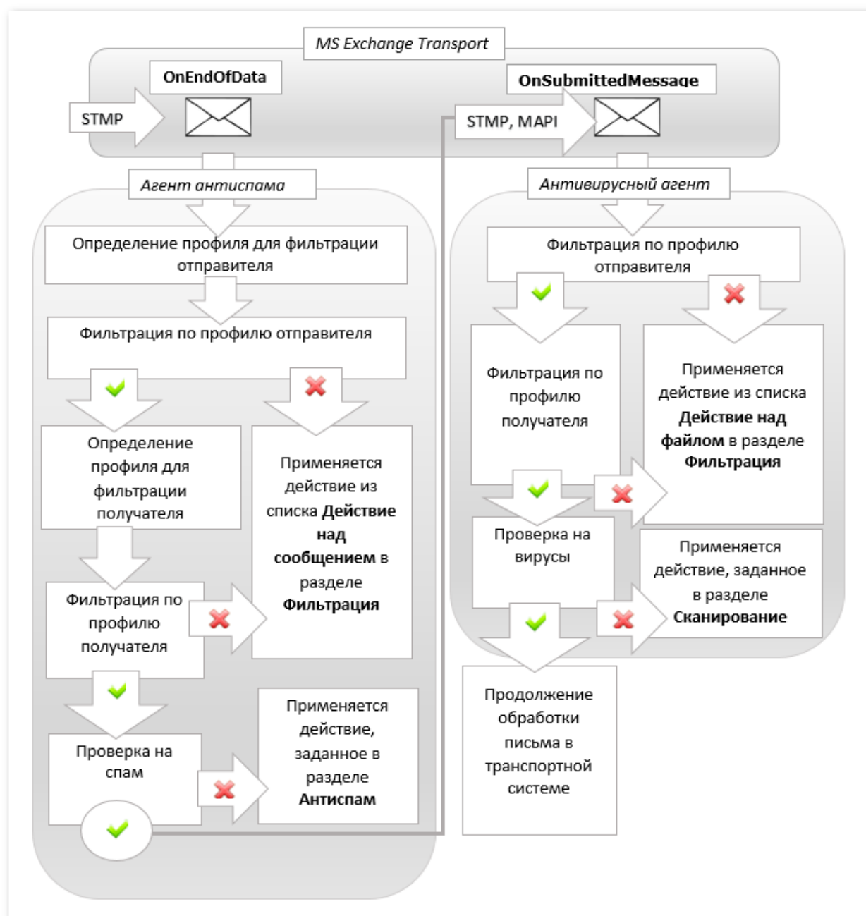
Рисунок 8. Фильтрация писем в транспортной системе
