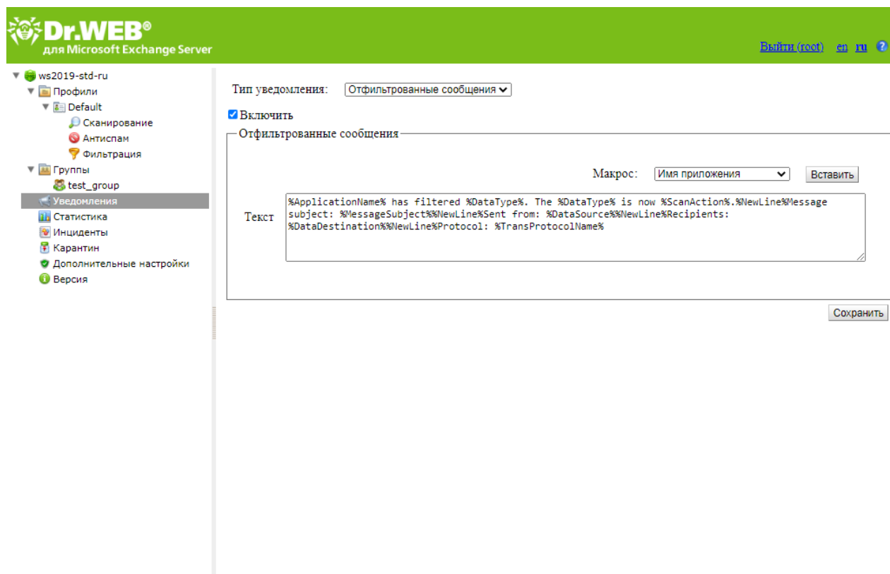
Рисунок 16. Раздел настройки уведомлений
