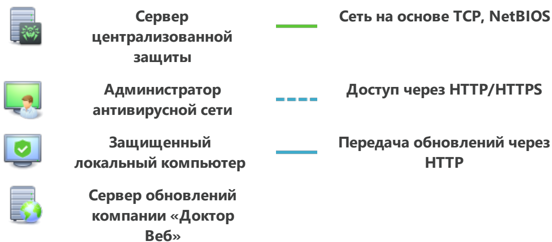
Рисунок 23. Логическая структура антивирусной сети
