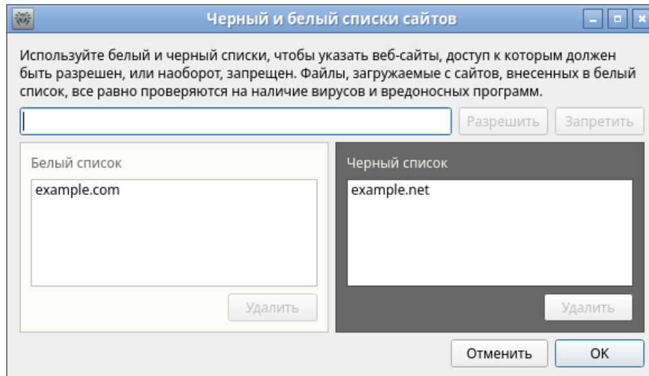
Рисунок 45. Окно управления черным и белым списками
