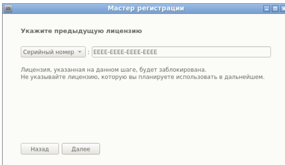
Рисунок 25. Указание предыдущей лицензии
