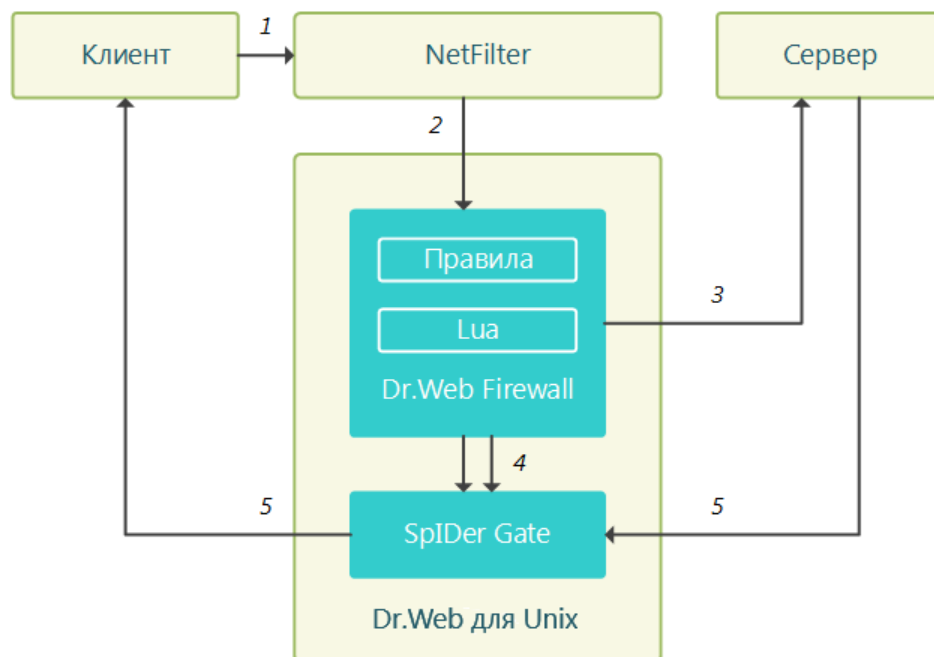
Рисунок 52. Схема работы Dr.Web Firewall для Linux
