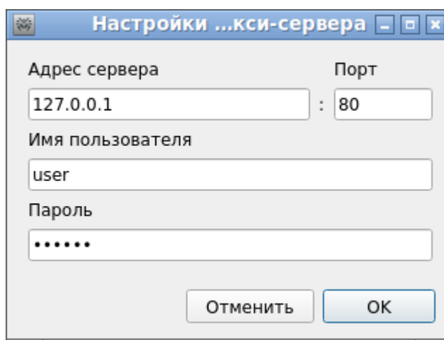
Рисунок 31. Настройки прокси-сервера
