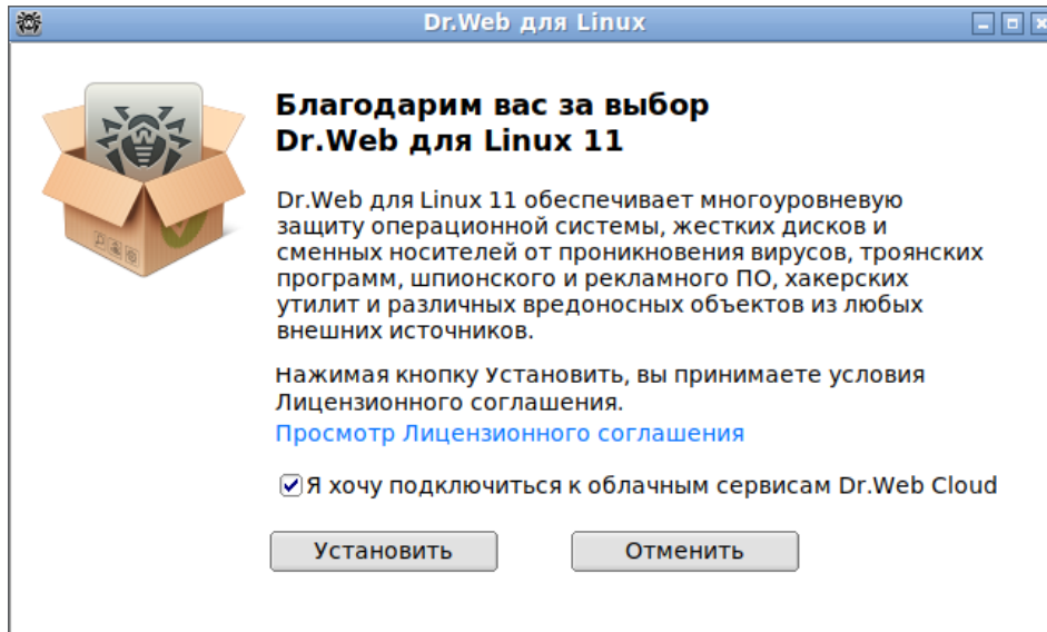
Рисунок 2. Мастер установки
