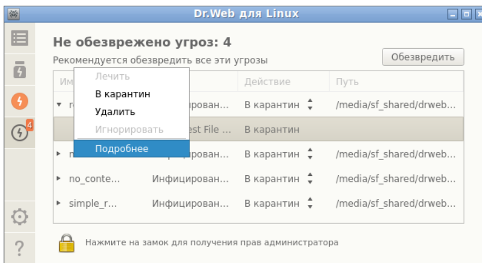
Рисунок 15. Обзор угроз
