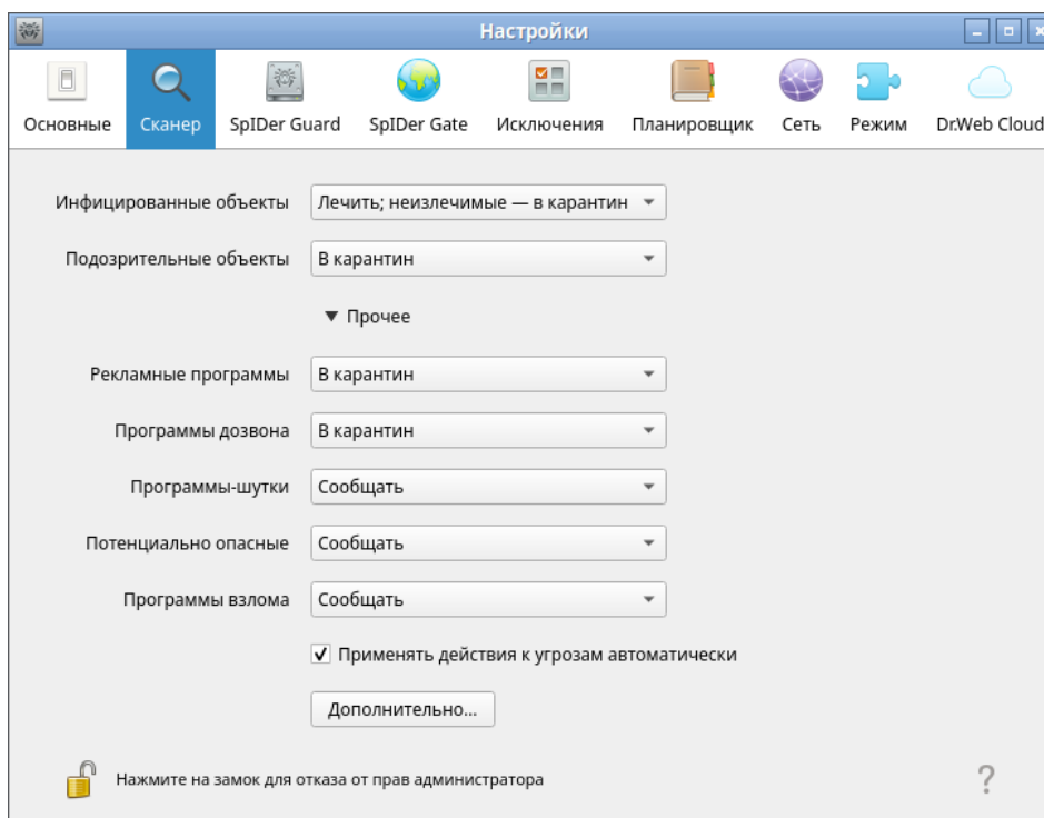
Рисунок 38. Настройки Сканера
