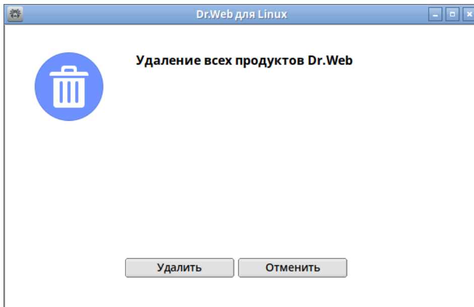
Рисунок 3. Мастер удаления
