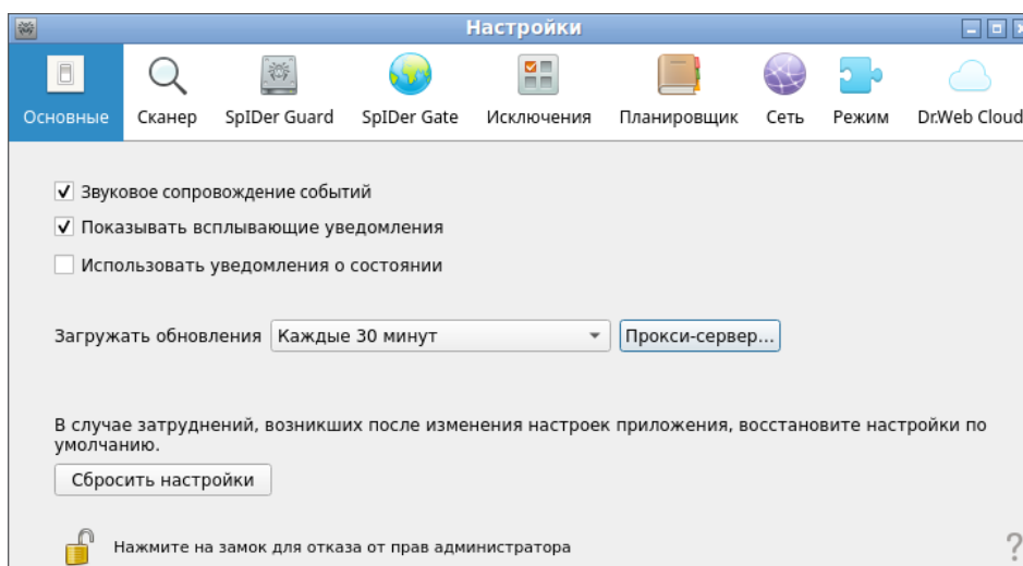
Рисунок 36. Основные настройки
