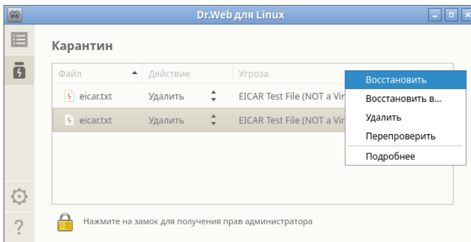
Рисунок 17. Управление карантином
