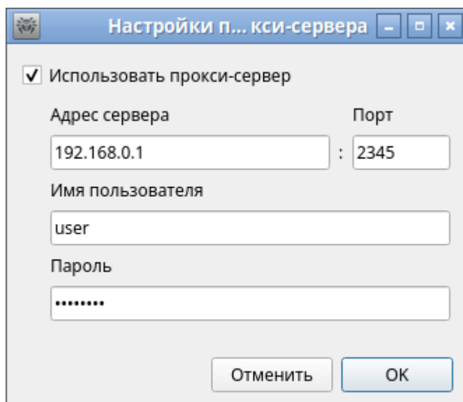
Рисунок 37. Настройки прокси-сервера
