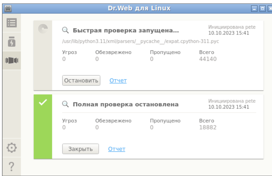
Рисунок 11. Список проверок
