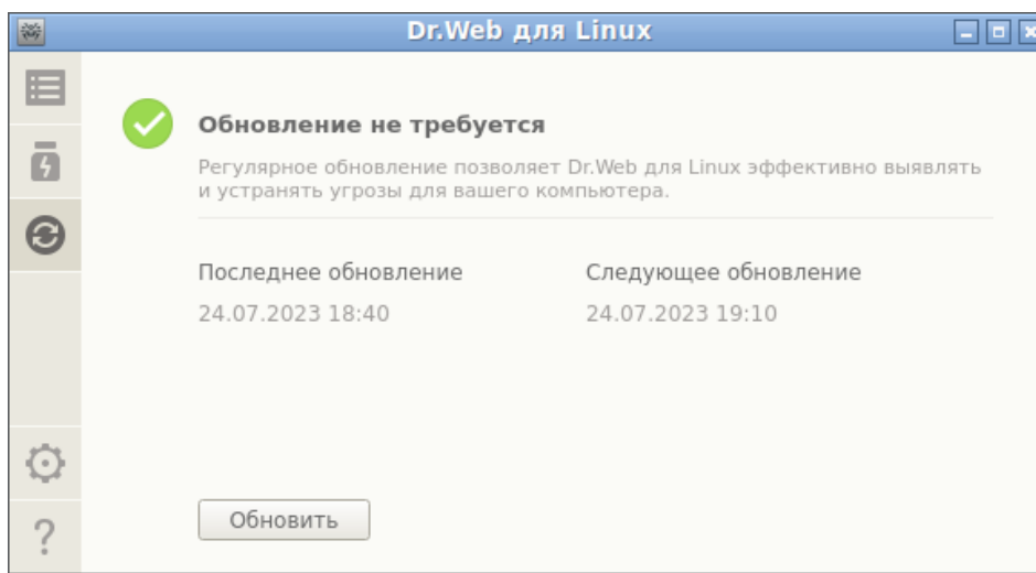
Рисунок 19. Управление обновлением
