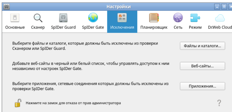
Рисунок 43. Настройка исключений
